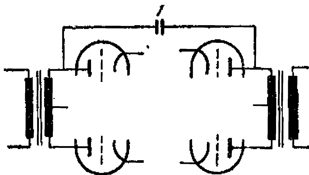
Fig. II.62. Sincronizarea a două oscilatoare cu ajutorul unei capacități C .
