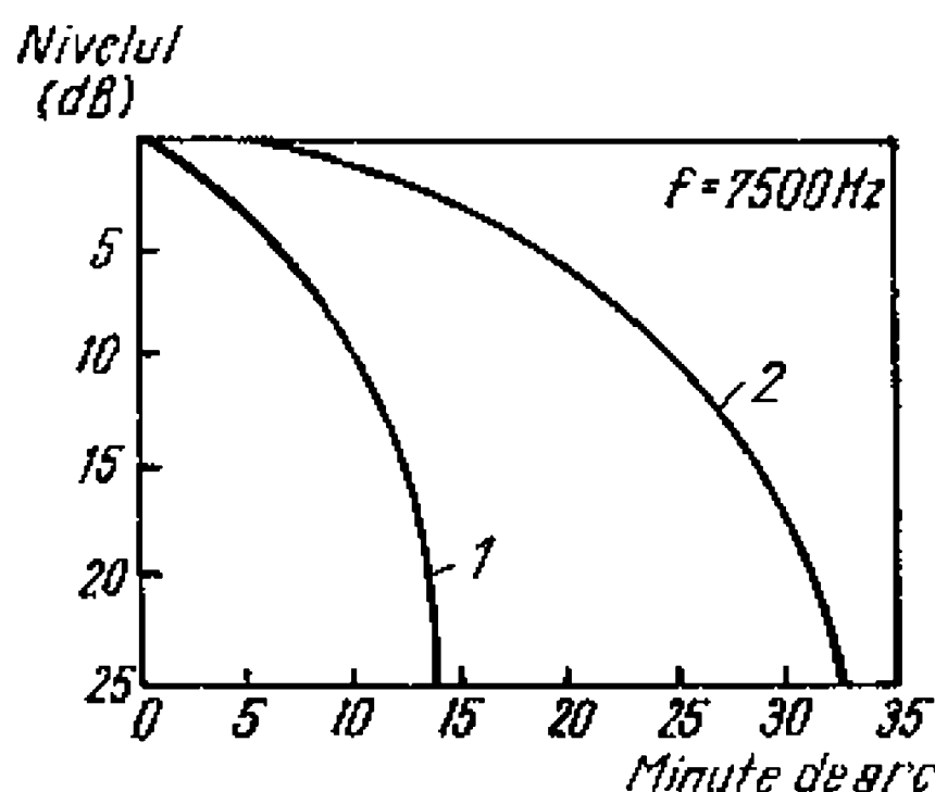
Fig. II.69. Pierderi într-un cap de redare datorită nealinierei fantelor:
