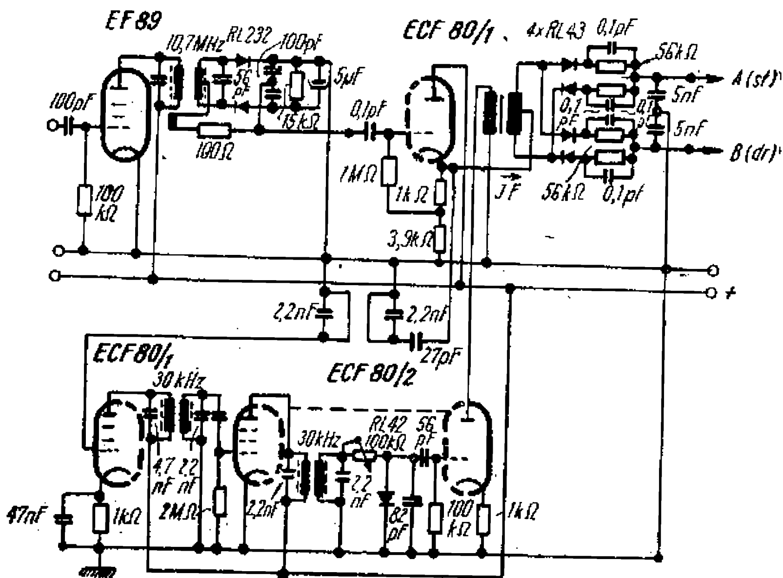
Fig. IV.45. Adaptor stereofonic după procedeul PAM.
