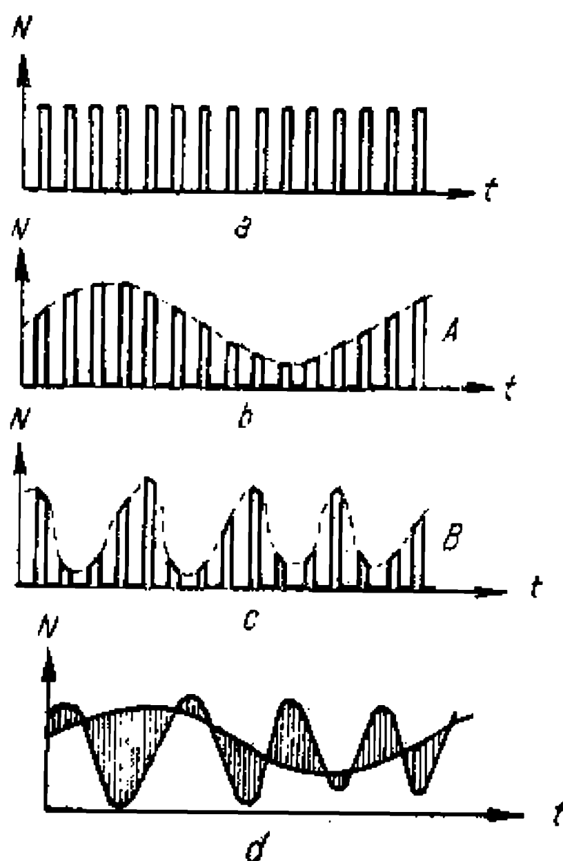
Fig. IV.35. Sistemul multiplex prin impulsuri de amplitudine modulată.
