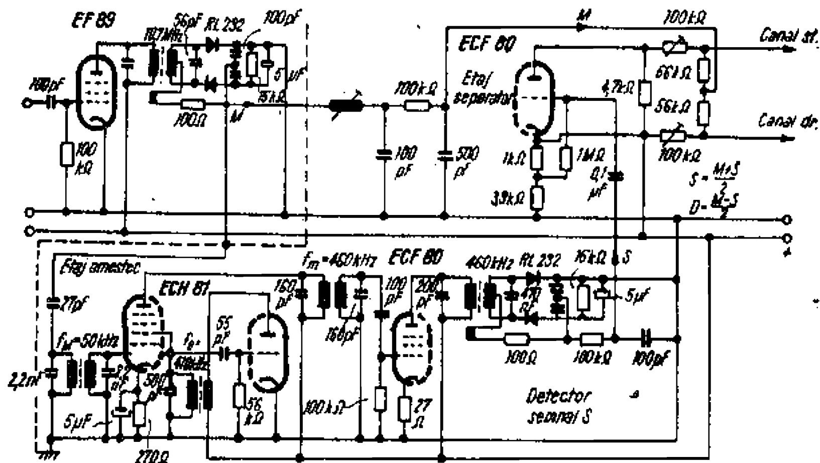
Fig. IV.41. Adapter la radioreceptor folosind procedul multiplex prin curenți purtători.
