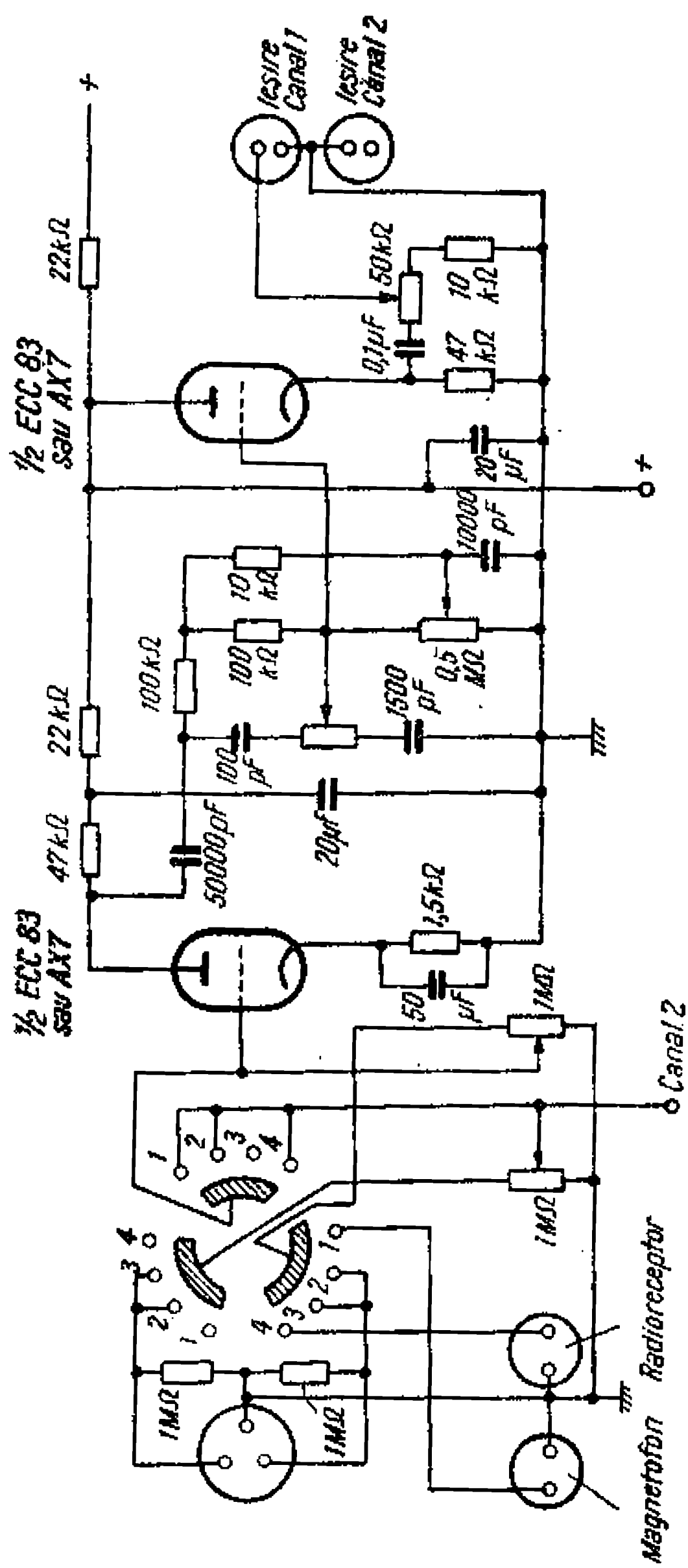
Fig. II.59. Preamplificator pentru adaptarea agregatului de redat discuri monofonice.
